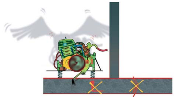
On supprime la propagation solidienne en « suspendant » la machine sur des liaisons souples : c'est l'isolation vibratoire.
