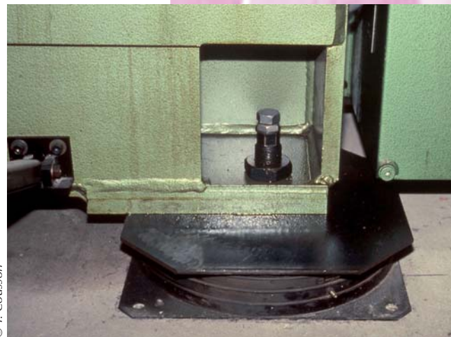
Exemple de suspension élastique
